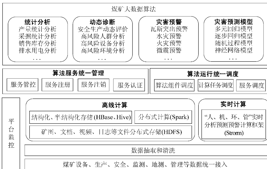
图2 煤矿安全生产大数据分析平台技术框架
