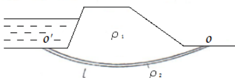
图D.1 堤坝底部渗漏模型示意图
